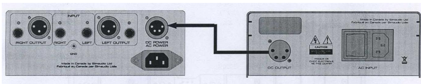
Рисунок 2 : Задняя панель “Moon 310LP” и “Moon 320S”.
